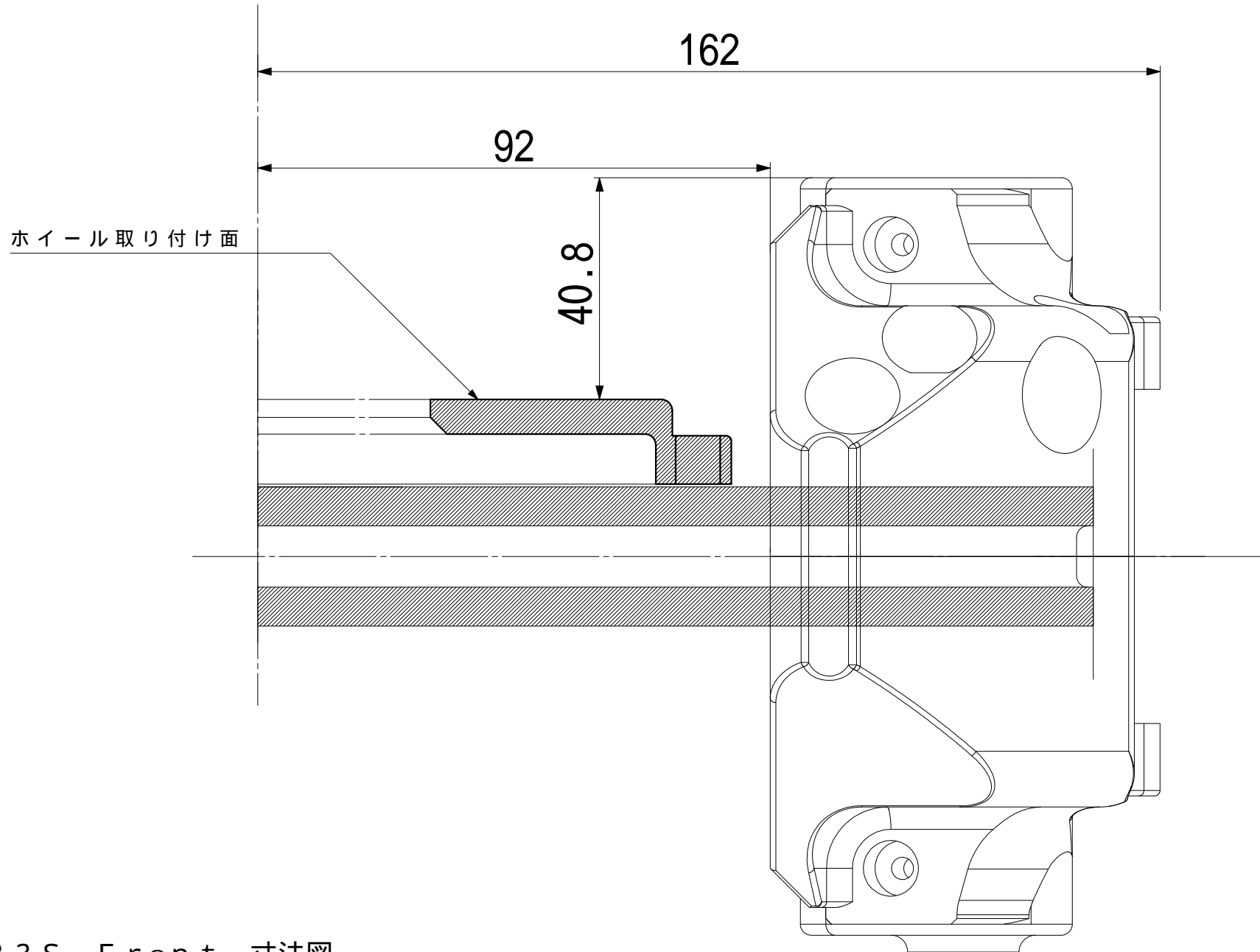
ZC33S Front 寸法図
